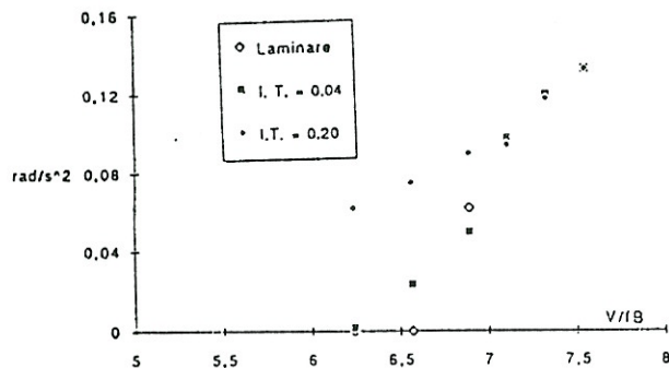
Fig. 7: Simulazione analitica: andamento dell'R.M.S. della accelerazione torsionale nel caso di instabilità da flutter
