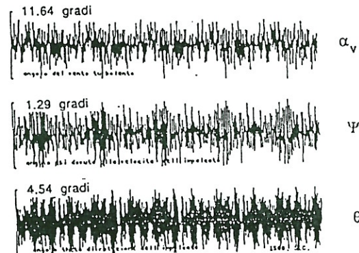
Fig. 8: Andamento temporale delle tre componenti dell'angolo di incidenza istantaneo per instabilità tipo flutter
