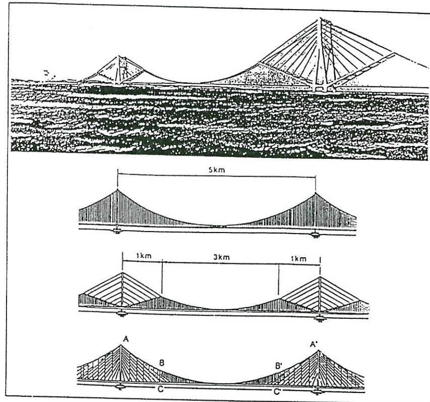
Fig 3, Progetto del ponte sullo stretto di Gibilterra
