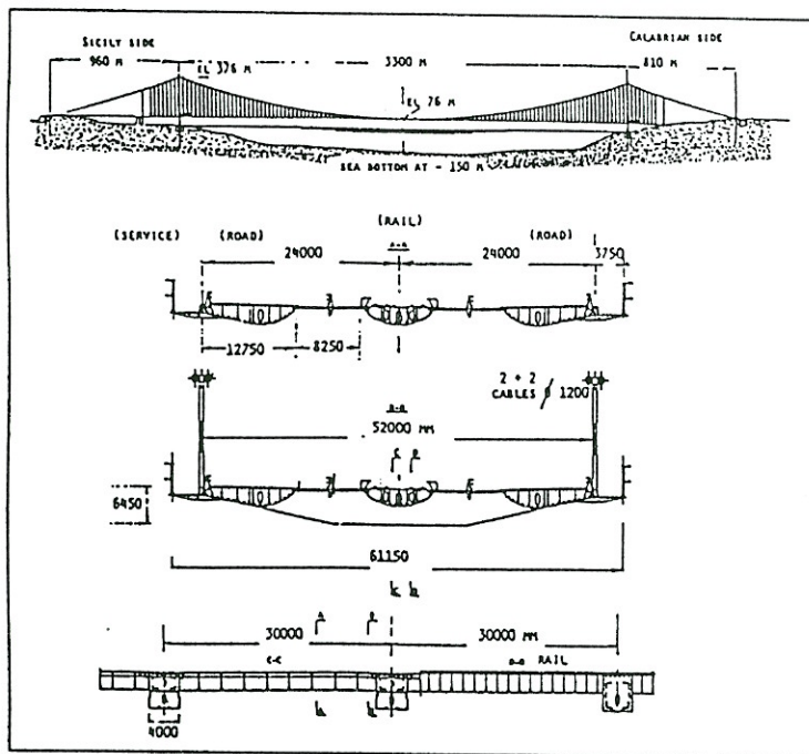
Fig 2, Progetto del ponte sullo stretto di Messina
