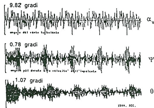
Fig. 6: Andamento temporale delle tre componenti dell'angolo di incidenza istantaneo per instabilità torsionale.
