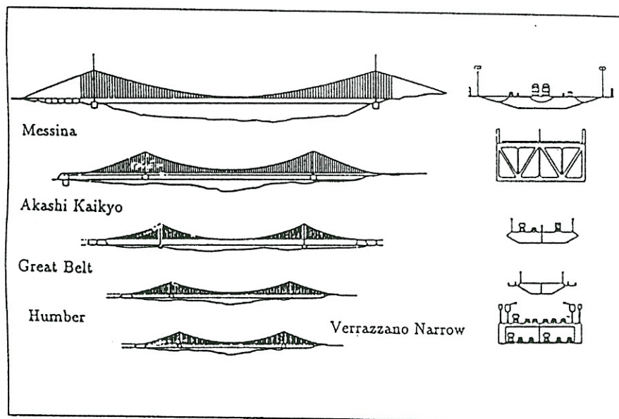
Fig. 1, Evoluzione dei ponti sospesi di grande luce
